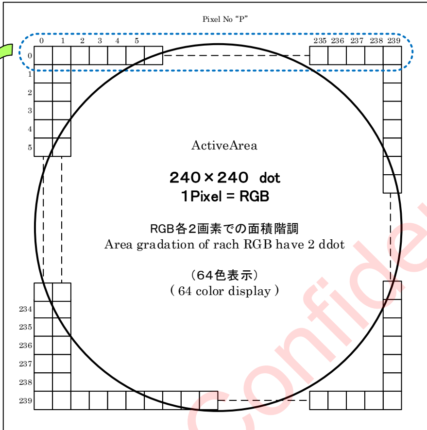
1Line分のピクセルデータと画素比率について About Pixel data of 1 line and the area ratio of 1 pixel.
